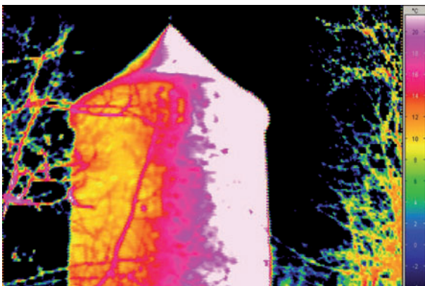
Bild 23: Wärmebildaufnahme eines Altstadtturms an einem Februartag um 17 Uhr. Die Sonne schien den ganzen Tag.
