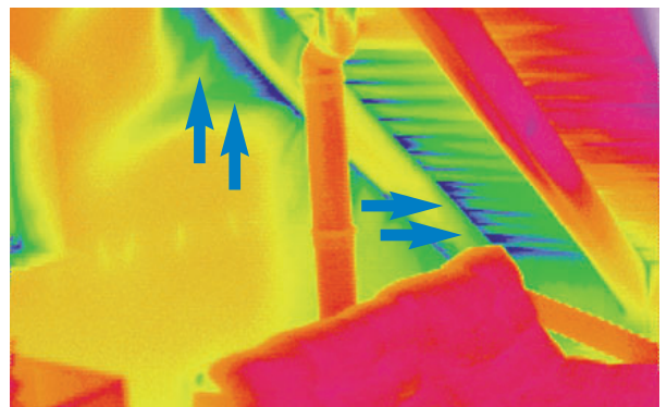
Bild 8: Wärmebildaufnahme dieser Wohnung
